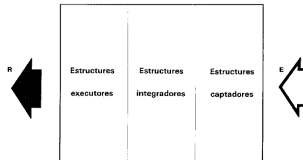
Fig. 2-1. Diagrama dels components bàsics de tot sistema nerviós animal.
